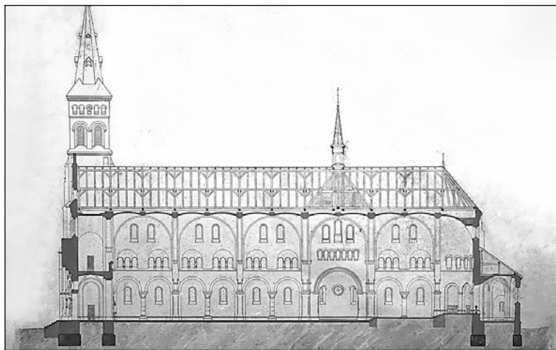
Projekt błażowskiego kościoła.
